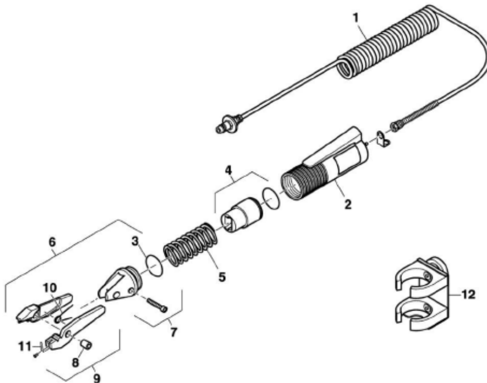
Рисунок 6 Запасные части
